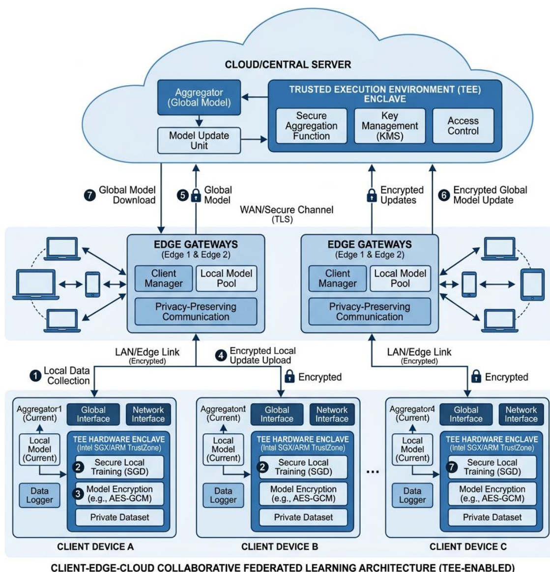
图 1: 联邦计算网络交互: 基于 TEE 锚点加密的端边云协同物理架构图
